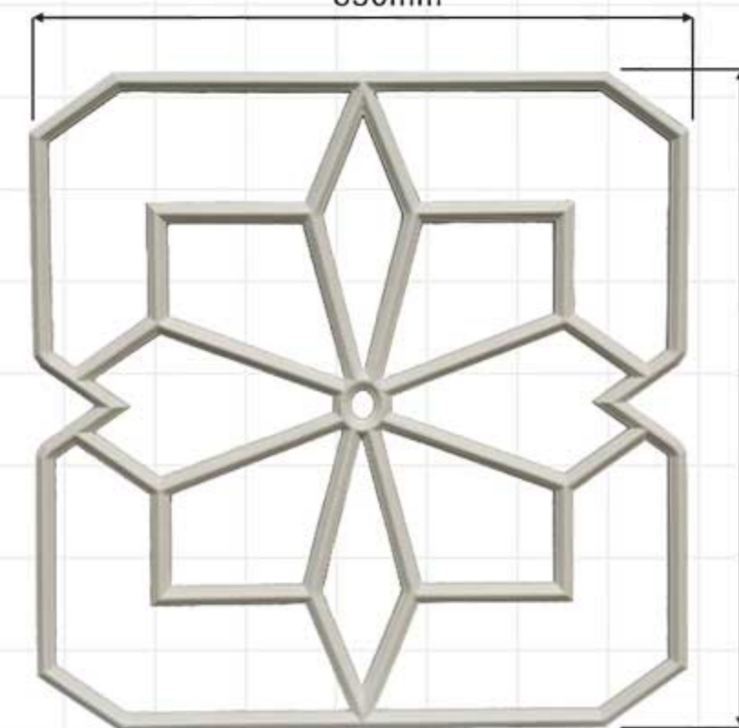
M-7411 D:850x850x20mm
