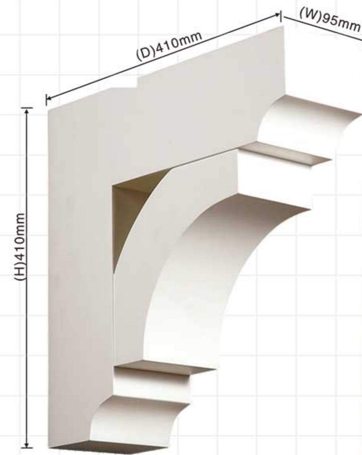
GL-6045 (H)410x(W)95x(D)410mm
